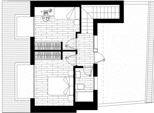
Planta Ático
