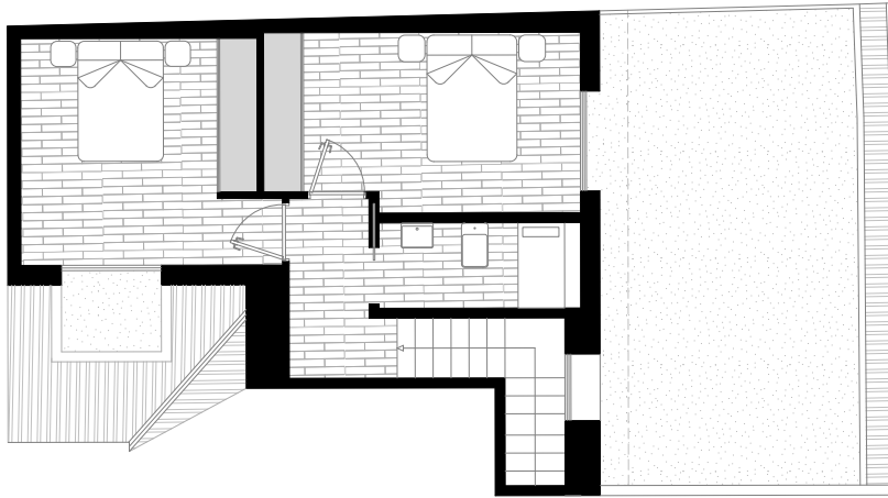
Planta Ático
