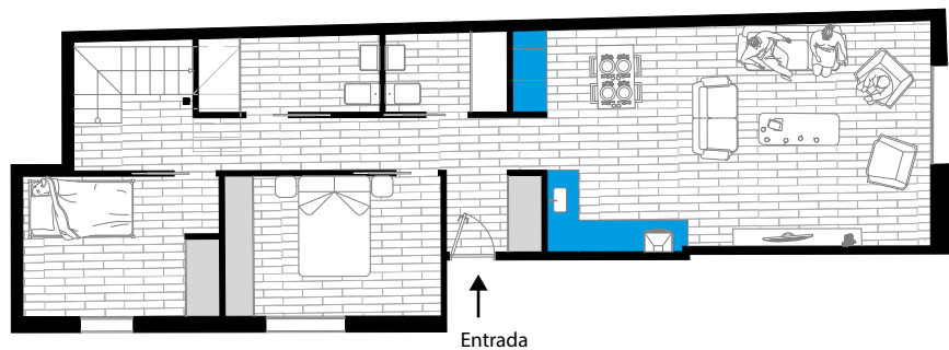
Planta Segunda
