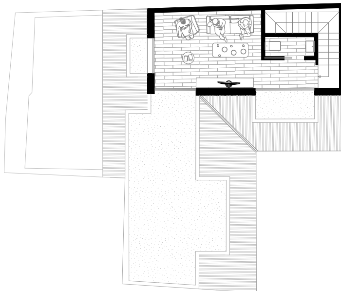
Planta Ático
